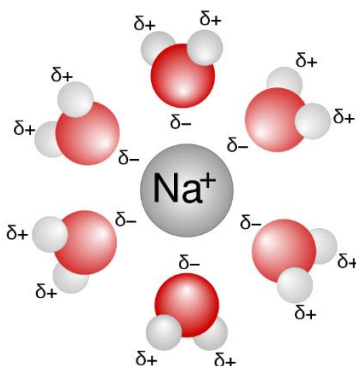
Gambar 7. Ion-Ion Disolvasi Dalam Larutan NaCl. Ion Positif Berinteraksi Dengan Oksigen Air Dan Ion Negatif Berinteraksi Dengan Hidrogen Air
