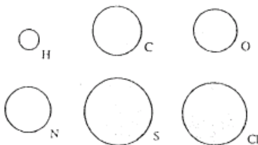
Gambar 1. Ukuran Relatif Atom H, C, O, N, S Dan Cl
